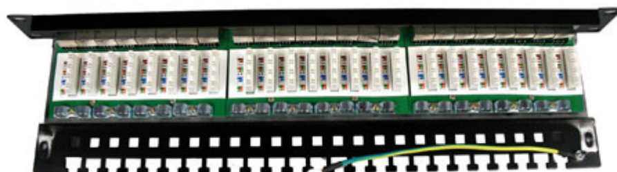
Horní pohled, konektory, zadní vyvazovací lišta a upínání kabeláže
